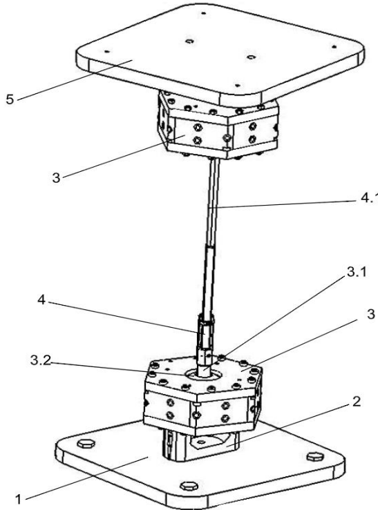
Şekil: Yedi serbestlik dereceli manipülatör sisteminin üst tabla yerleştirilmiş izometri görünümü
